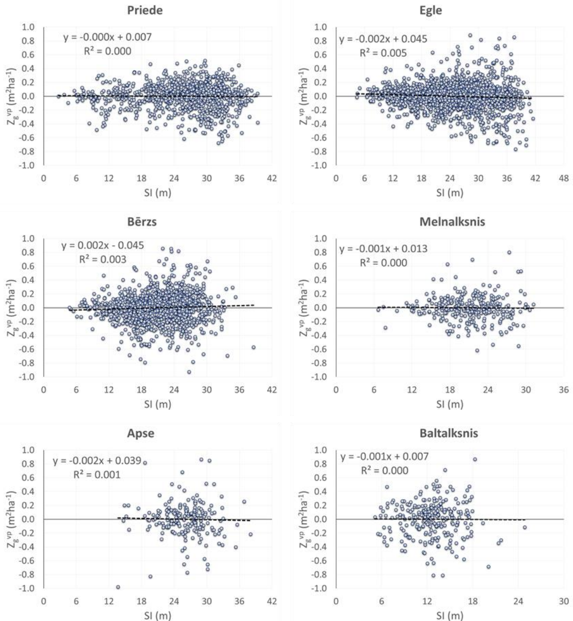
2.23. attēls. Starpība starp uzņēmīto un prognozēto meža elementa šķērslaukuma vidējo periodisko pieaugumu ( z_g^{vp} ) atkarībā meža elementa augstuma bāzes vecumā jeb bonitātes (SI).
