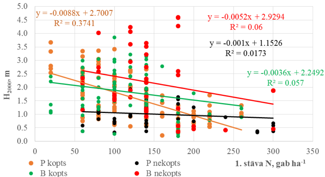
5.1. attēls. Piecu augstāko priežu vai bērzu uzskaites laukumā jeb 2000 kociņu uz ha vidējais augstums ( H_{2000} ) Ln 10 gadus pēc ciršanas atkarībā no audzes 1. stāva koku skaita koptās un nekoptās jaunaudzēs
