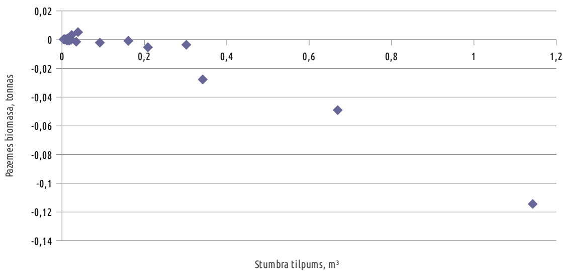
24. Attēls: Atlikumu izklīde egles celma un sakņu biomasas aprēķinam.
