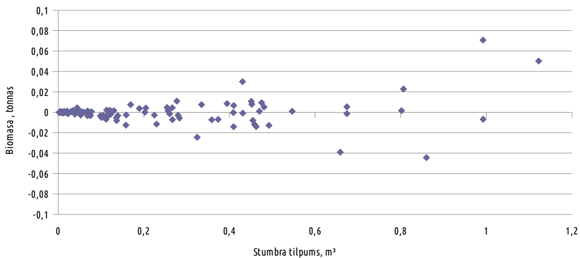
4. Attēls: Atlikumu izkliede bērza virszemes biomasas aprēķinam.
