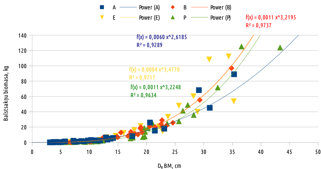
29. Attēls: Baltsakņu biomasas un celma caurmēra sakarība.
