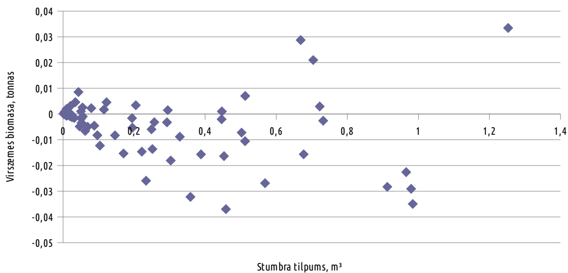
10. Attēls: Atlikumu izkliede apses virszemes biomasas aprēķinam.
