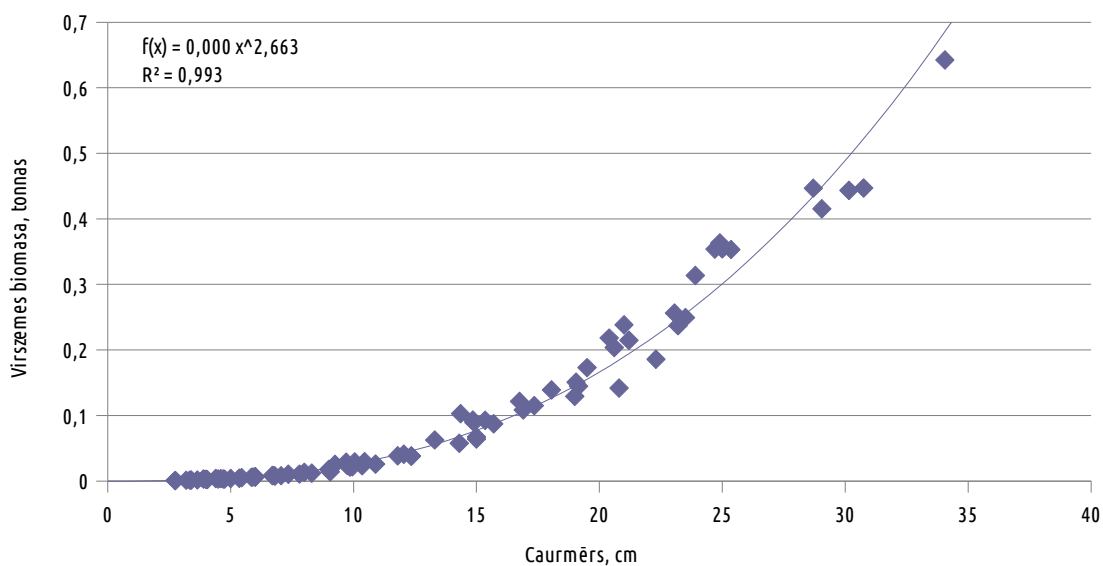
13. Attēls: Apses virszemes biomasas atkarībā no koka krūšaugstuma caurmēra.
