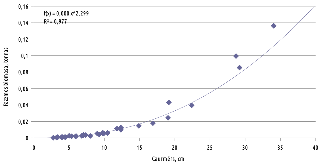
14. Attēls: Apses celma un sakņu biomasā atkarībā no koka krūšaugstuma caurmēra.
