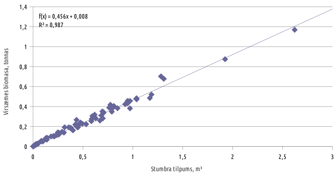
15. Attēls: Stumbrā tilpuma un virszemes biomasas attiecība priedei.
